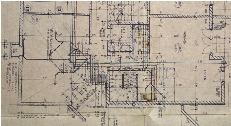
Grundriss Erdgeschoss, Ablauffleitungen in Decke Erdgeschoss bzw. Boden 1. Stock / IMG_5493.jpg
