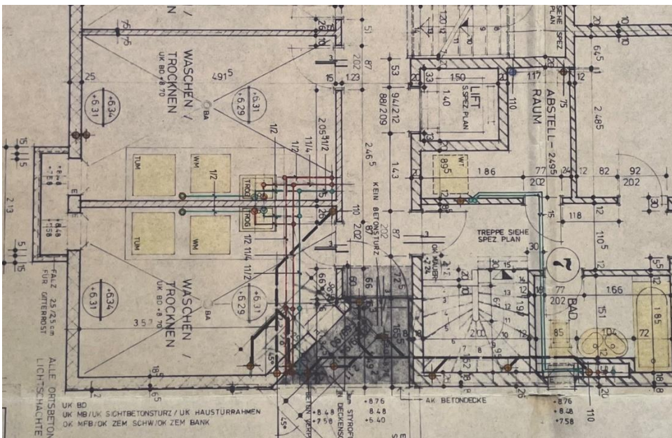
Grundriss 1. Stock, Ablauffleitungen in Decke 1. Stock bzw. Boden 2. Stock / 1.St_Wo_7_IMG_5496_A.jpg
